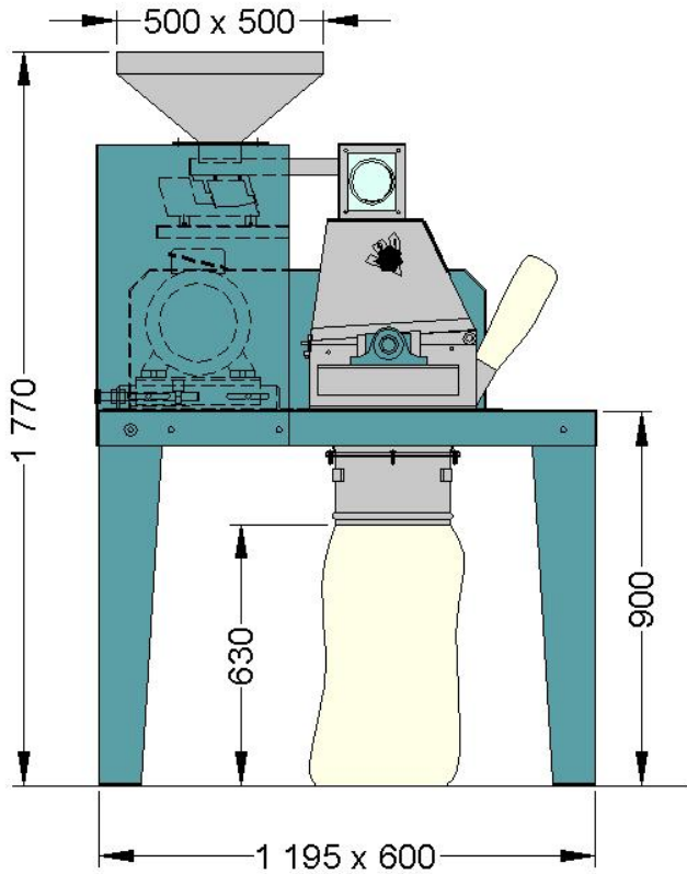
F3 avec distributeur vibrant
