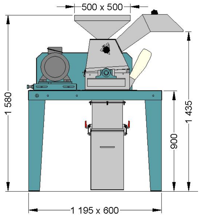
F3 avec goulotte d'alimentation
